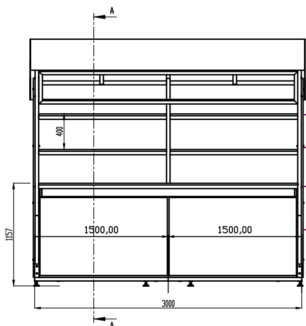
Prospetto disegno tecnico quotato
