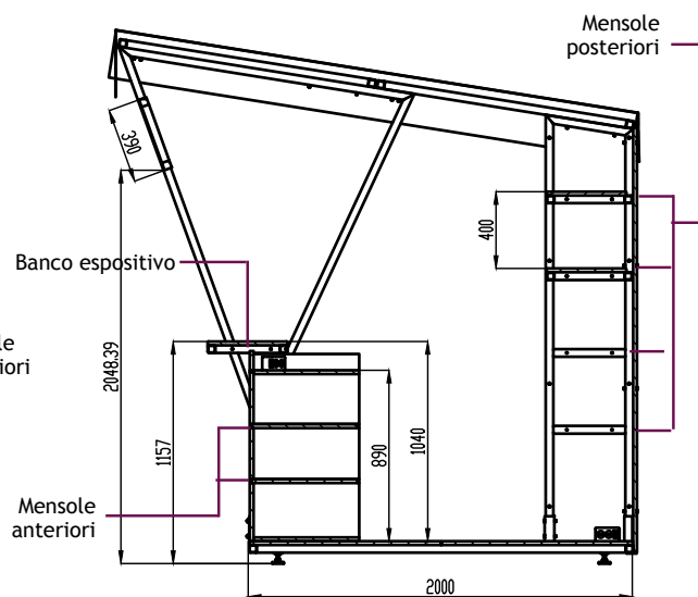
Sezione disegno tecnico quotato
